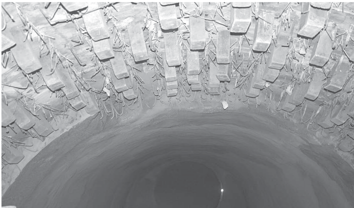
Монтаж футеровки внутри печи прокаливания С-3421
