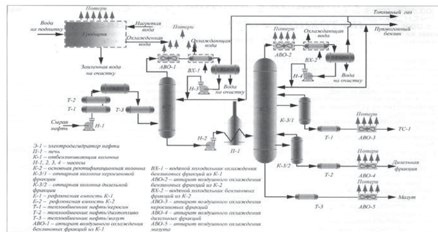
Рис. 1. Типовая принципиальная схема установки ЭЛОУ-АТ
