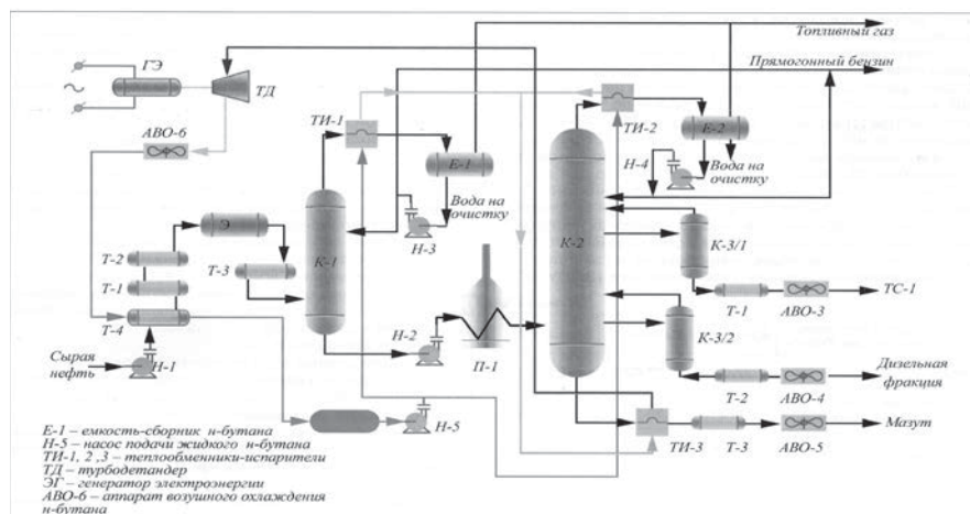
Рис. 2. Принципиальная схема установки ЭЛОУ-АТ с генерацией электроэнергии
