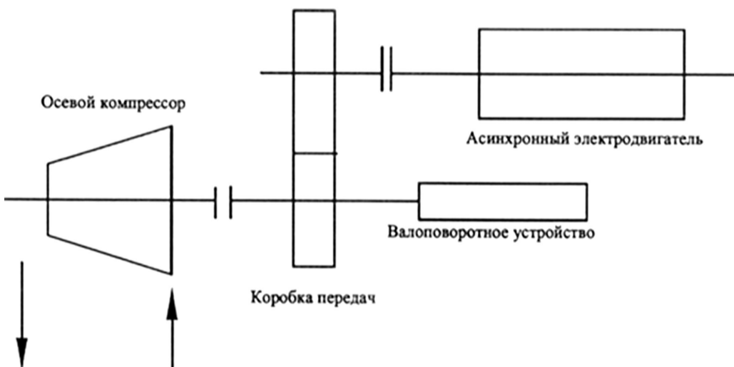
Схема осевого компрессора Осевой компрессор K-0101 модели AV71-13 имеет 13 ступеней, которые образуются статическими и динамическими лопатками. Диаметр ступицы ротора осевого компрессора – 710
