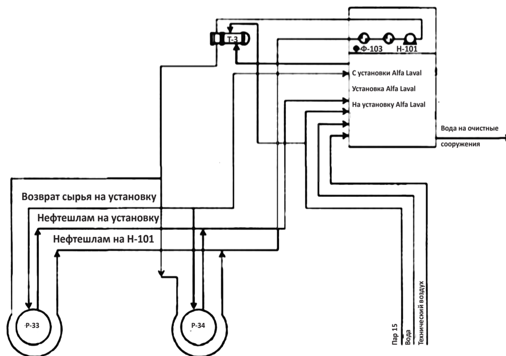
РИСУНОК 1 – ТЕХНОЛОГИЧЕСКАЯ СХЕМА УТИЛИЗАЦИИ НЕФТШЛАМА
