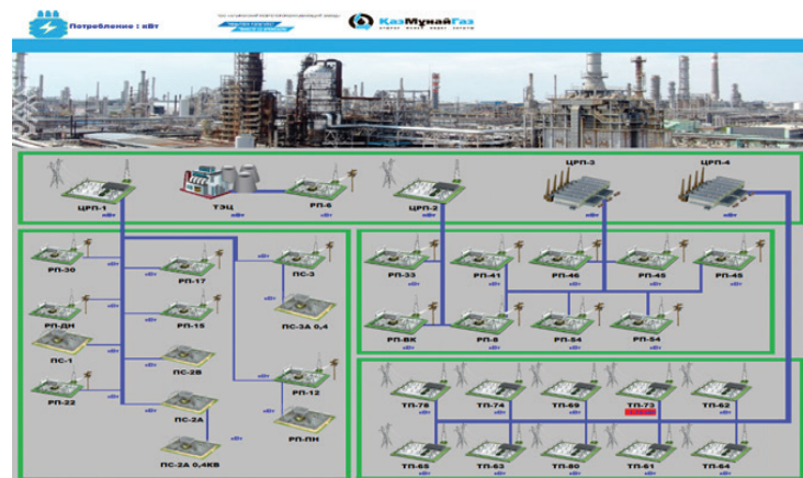
Рис 1. Структурная схема технологического процесса
